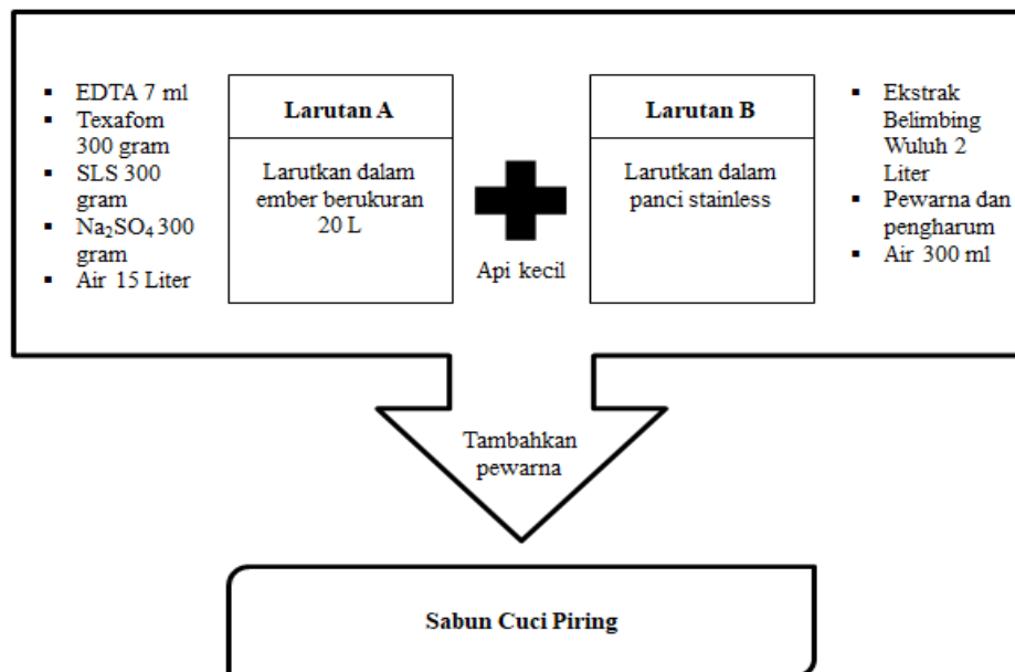
Gambar 1. Diagram alir pembuatan sabun cuci piring
